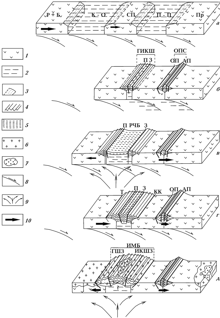
Рис. 3. Упрощенная внемасштабная схема предполагаемого палеогеодинамического процесса в центральной и восточной частях УЩ (стадии процесса (а–д) объясняются в тексте): 1 — континентальные микроплиты, состоящие из архейских мегаблоков (Р + Б — Росинского и Бугского, СП — Среднеприднепровского, Пр — Приазовского); 2 — океанические (субокеанические) микроплиты (К-О — Криворожско-Одесская, П-П — Приднепровско-Приазовская); 3 — терригенно-вулканогенно-карбонатные толщи, откладываемые на континентальных окраинах (геоклиналях); 4 — складчатость в породах коллизионных швов; 5 — вулканогенно-осадочные образования Рощаховско-Чечелеевского бассейна; 6–7 — протерозойская гранитизация архейских мегаблоков (6 — 2,0 + 2,1 млрд лет назад, 7 — 1,75 + 1,8 млрд лет назад); 8–9 — направление движения мантийного вещества (8 — в восточной ветви конвективной ячейки или мантийного плюма регионального масштаба, 9 — в пульсирующем мантийном плюме местного масштаба); 10 — направление перемещения континентальных плит (длина стрелки отражает условную относительную скорость перемещения плиты). ГИКШ — Головановско-Ингулецко-Криворожский коллизионный шов, ОПС — Орехово-Павлоградская сутура, РЧБ — Рощаховско-Чечелеевский бассейн, ИМБ — Ингульский мегаблок, ГШЗ — Головановская шовная зона, ИКШЗ — Ингулецко-Криворожская шовная зона. Зоны разломов: П — Первомайская, З — Западно-Ингулецкая, ОП — Орехово-Павлоградская, АП — Азовско-Павловская, Т — Тальновская, КК — Криворожско-Кременчугская.
