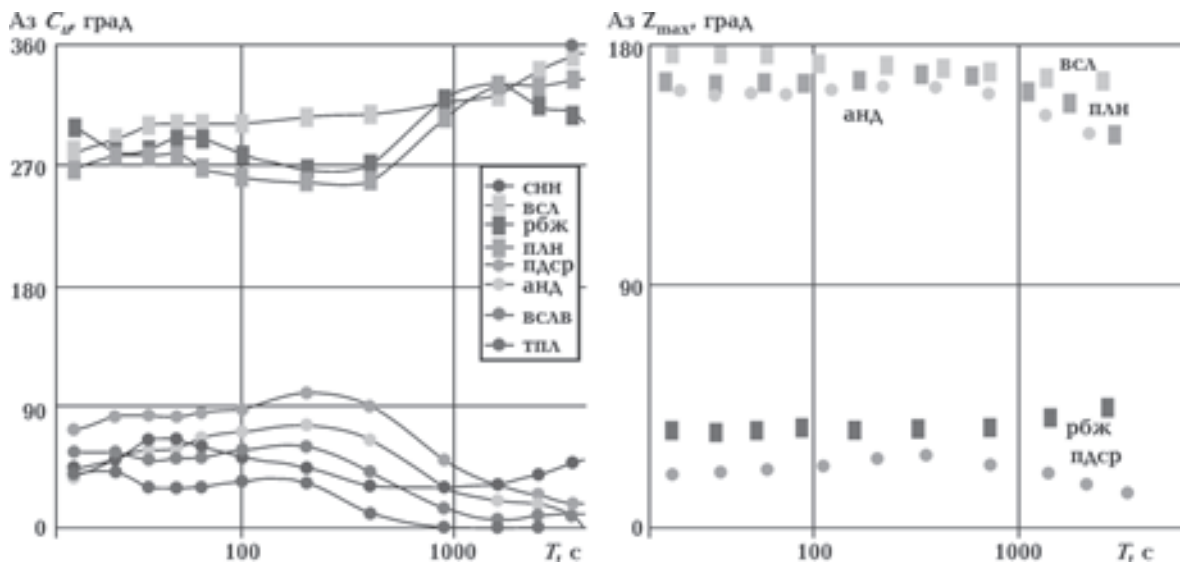
Рис. 2. Распределение AzC_u и AzZ_{max} вдоль профиля пр_аз110.
