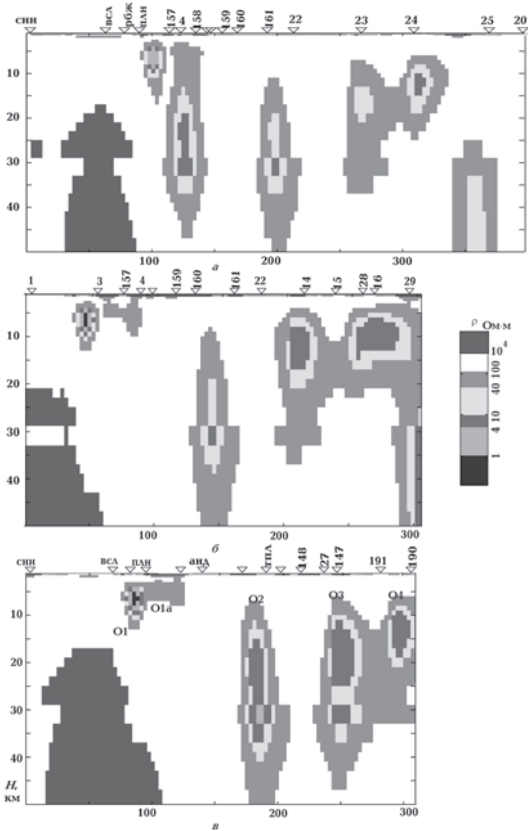
Рис. 3. Геоэлектрические модели вдоль интерпретационных профилей с различными азимутами: а — пр_аз70 (m13), б — пр_аз90 (m04), в — пр_аз110 (m06).
