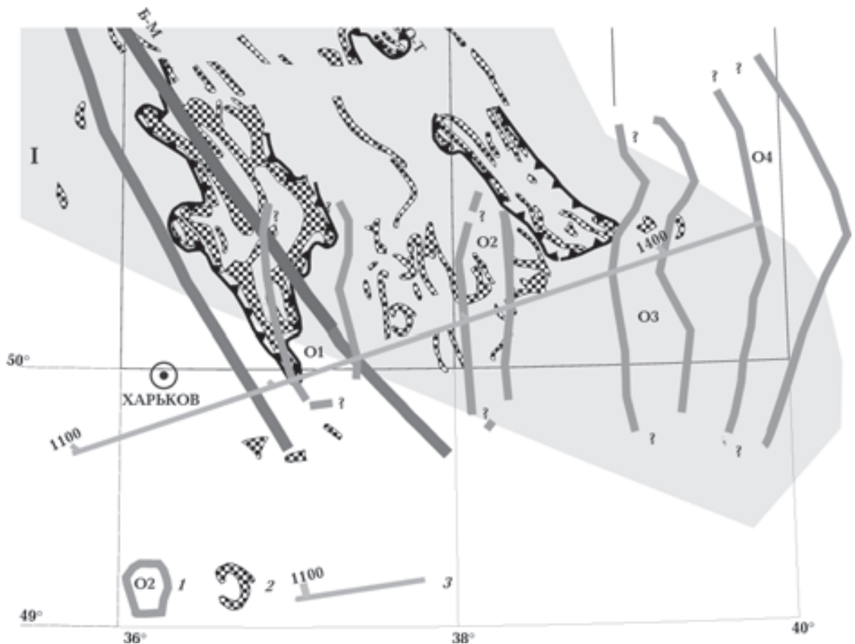
Рис. 4. Основные тектонические структуры ВКМ и объекты пониженного сопротивления (1), железистые кварциты (2) и положение геотраверса «Гранит» (3). Остальные обозначения см. на рис. 1.
