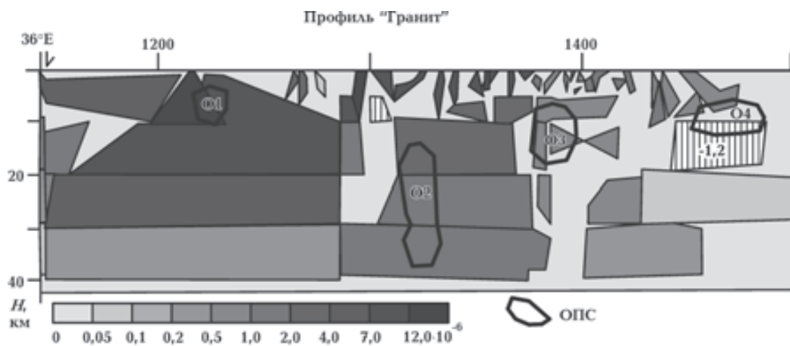
Рис. 5. Сопоставление объектов пониженного сопротивления с объектами магнитных аномалий.
