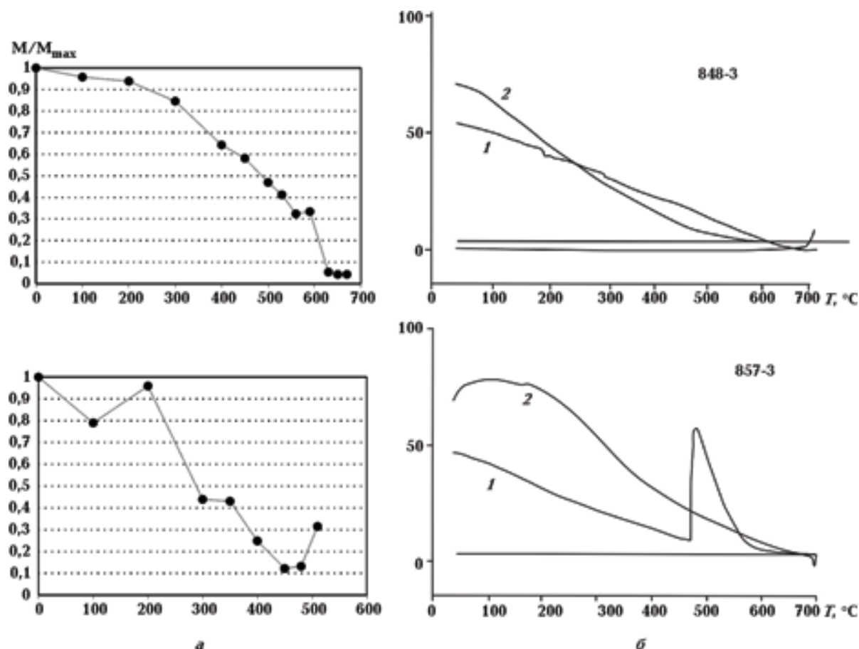
Рис. 6. Примеры разрушения: нормированной ЕОН в процессе ступенчатого терморазмагничивания (а); остаточной намагниченности насыщения в процессе непрерывного нагрева (1 — первый нагрев, 2 — второй нагрев) образцов коновской свиты верхнего силура (б).
