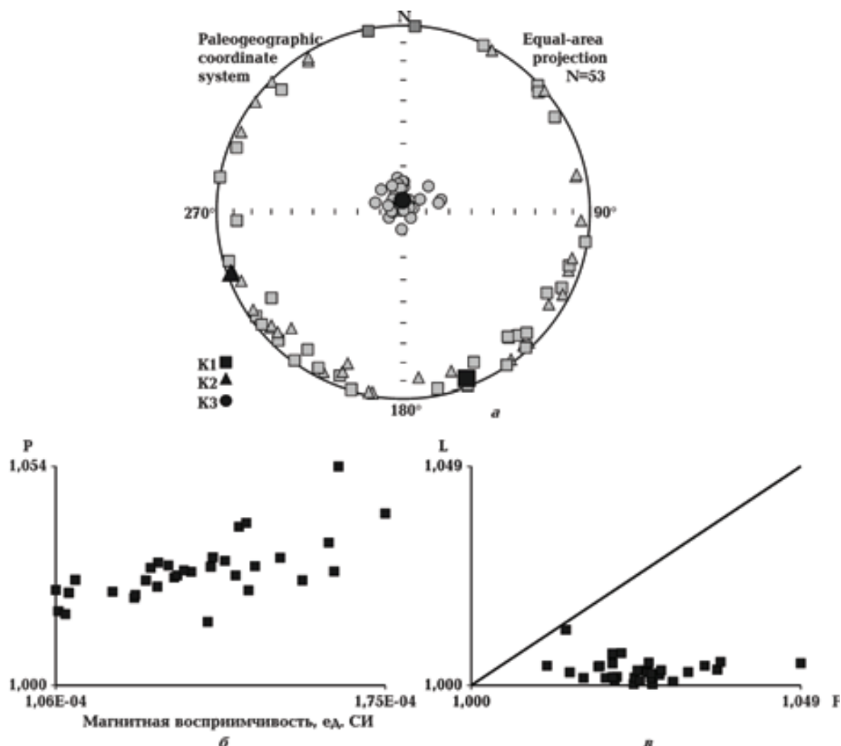
Рис. 7. Распределение осей эллипсоидов анизотропии магнитной восприимчивости (K1, K2 и K3 — средние направления соответственно максимальной, средней и минимальной осей (a); диаграмма степени анизотропии магнитной восприимчивости P = K1/K3 относительно величины магнитной восприимчивости (б); распределение отношений главных осей эллипсоидов АМВ на диаграмме Д. Флинна, L = K1/K2 , F = K2/K3 (в).
