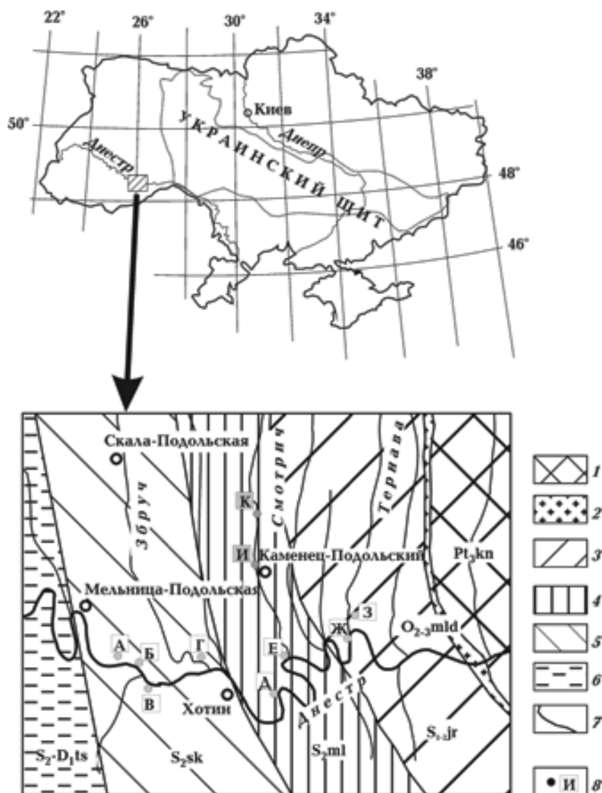
Рис. 2. Геологическая схема палеозоя среднего Приднестровья (со снятым мезо-кайнозойским чехлом). Исследованные разрезы силурийских пород (А—З) приведены в соответствии с маркировкой [Jeleńska et al., 2005], местоположение разрезов красноцветов силура обозначено буквами И и К: 1—6 — серии (1 — каниловская, 2 — молодовская, 3 — яругская, 4 — малиновецкая, 5 — скальская, 6 — цыганская), 7 — границы серий, 8 — исследованные обнажения.
