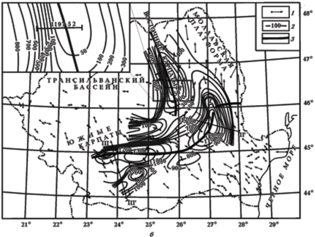
Рис. 8. Профили МТЗ на тектонической карте Румынии [Stanica et al., 1999] (а) и векторы Визе (б) для периодов 5—50 мин (1), изолинии суммарной продольной проводимости (в См) осадков по данным МТЗ (2) и ось КАЭ (3). На врезке сверху расположение детального профиля и пункты над осевой зоной КАЭ, кривые в которых даны на рис. 7, г. [Pinna et al., 1992].
