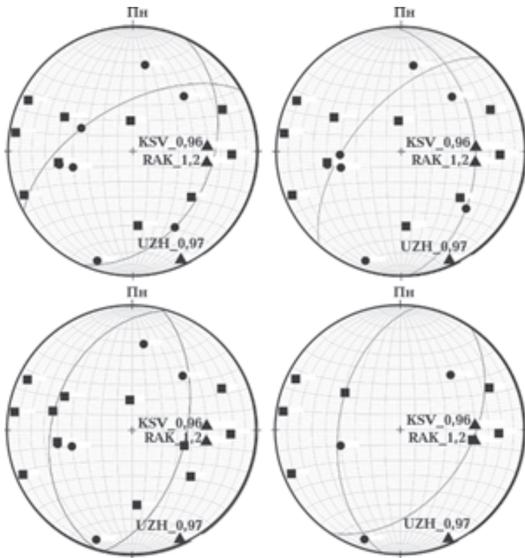
Рис. 7. Варіанти розміщення нодальних площин для події 15.11.2006, 18:09:38,5. Кругок — станції, на яких зафіксовано стиск, квадратик — розтяг, трикутник — нечіткі вступи. Білі станції з нечіткими вступами визначено логарифм відношення амплітуди S -хвилі до амплітуди P -хвилі.
