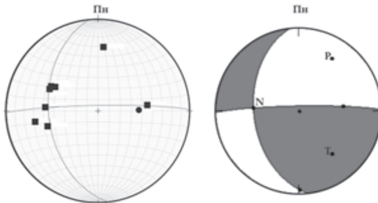
Рис. 23. Механізм вогнища землетрусу для події 04.04.2013.
