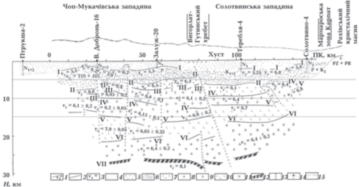
Рис. 5. Сейсмогеологічний розріз земної кори вздовж Закарпатського прогину: 1 — заломлюючі горизонти із зазначеними граничними швидкостями ( V_T ), 2 — відбиваючі горизонти і їх номери, 3 — пластова швидкість, 4 — неогенова моласа, 5 — вулканіти в осадовому чохла, 6 — мезозойсько-палеогенова складчаста основа прогину, 7 — палеозойський(?) метаморфізований фундамент, 8 — шар пониженої швидкості в середині «граніту», 9 — докембрійський(?) кристалічний комплекс, 10 — «базальтовий» шар, 11 — шар пониженої швидкості в основі земної кори, 12 — розділ Мохоровичича, 13 — розломи, 14 — бурові свердловини, 15 — крива \Delta g .
