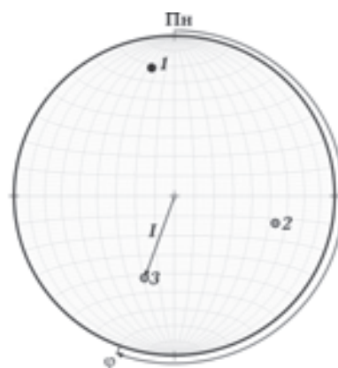
Рис. 4. Нанесення на стереографічну сітку точок — проєкцій променів: 1 — точки, що відповідають за нечіткий знак вступу; 2 — те саме, за полярність вступу P -хвилі зі знаком «+»; 3 — те саме, за полярність вступу P -хвилі зі знаком «-».
