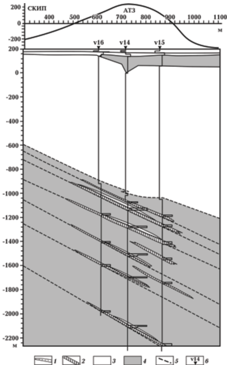
Рис. 5. Вертикальный разрез геоэлектрической аномальной зоны типа "залежь", по [Левашов и др., 2010]: 1, 2 — аномально поляризованный пласт (1 — типа "газ", 2 — типа "конденсат"), 3 — граниты, 4 — Na-метасоматиты, 5 — зоны дробления, 6 — пункты вертикального электрорезонансного зондирования.
