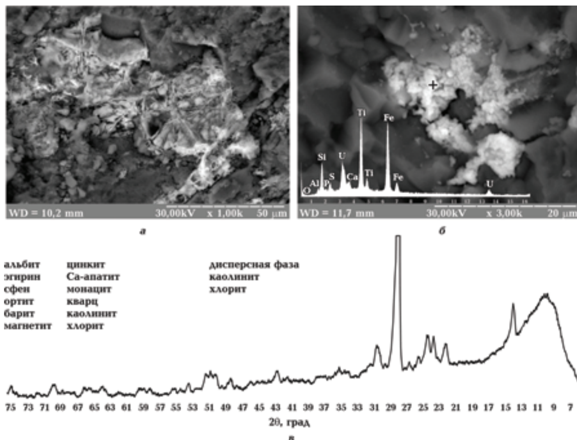
Рис. 3. Структура (а), характер урановой минерализации (б) и типичная дифрактограмма (в) ураноносных Na-метасоматитов Новокопастинской рудной зоны (а, б — электронный микроскоп РЭМ-106 с рентгеноспектральным анализатором, ЧО УкрГГРИ; в — ДРОН-3, Cu-антикатоде, Ni-фильтр, ЧО УкрГГРИ) (по А. Е. Лукину).
