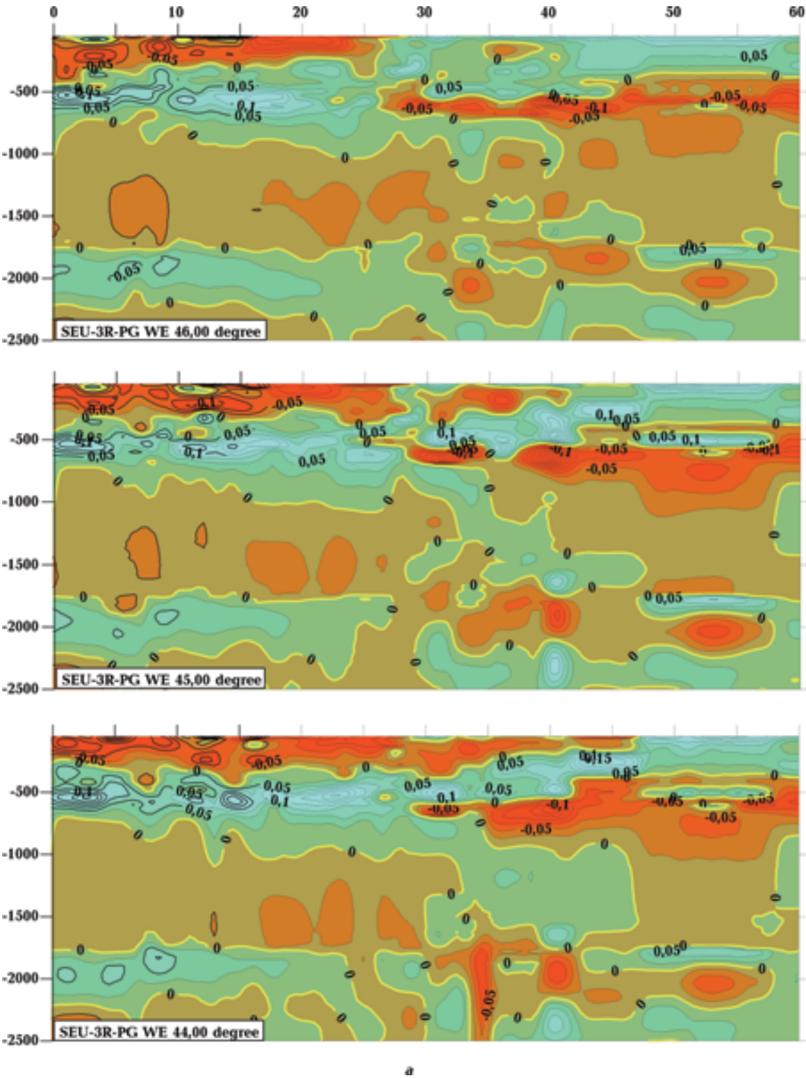
Рис. 6. Широтные сечения трехмерной P -скоростной модели мантии: а — 44 \div 46^\circ с. ш., б — 47 \div 49^\circ с. ш. (красным цветом показаны низкие скорости, синим — высокие, желтым — нулевая изолиния).
