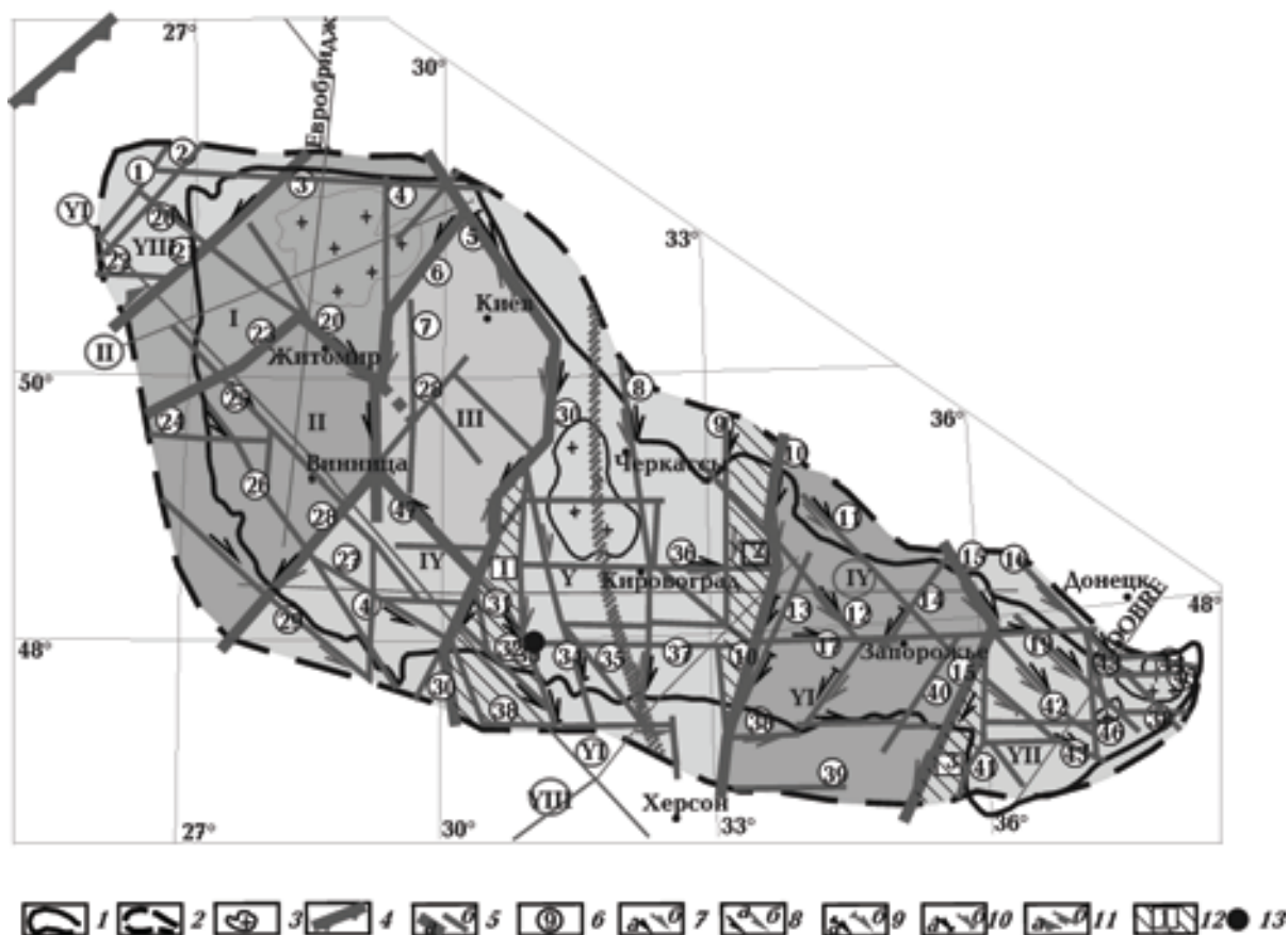
Рис. 1 Тектоническая схема и схема основных зон разломов УЩ и его склонов, по [Гинтов, Пашкевич, 2010]: 1 — контур обнаженной части щита, 2 — контур склонов щита, в пределах которых прослеживаются складчатые и разрывные структуры докембрийского фундамента по геофизическим данным, 3 — плутоны и крупные интрузивные массивы гранитоидов, 4 — граница между Сарматией и Фенноскандией, 5 — зоны разломов мегаблоковые (а), внутримергаблоковые (б), 6 — номера зон разломов (1 — Горынская, 2 — Луцкая, 3 — Полесская, 4 — Звиздаль-Залеская, 5 — Ядлов-Трактемировская, 6 — Чернобыльская, 7 — Брусиловская, 8 — Кировоградская, 9 — Западно-Ингулецкая, 10 — Криворожско-Кременчугская, 11 — Днепродзержинская, 12 — Светловодская, 13 — Саксаганская, 14 — Дерезоватская, 15 — Орехово-Павлоградская, 16 — Центрально-Волновахская, 17 — Девладовская, 18 — Малоянисольская, 19 — Краснополянская, 20 — Сарненско-Варваровская, 21 — Суцано-Пержанская, 22 — Владимир-Волынская, 23 — Тетеревская, 24 — Хмельницкая, 25 — Хмельникская, 26 — Летичевская, 27 — Ободовская, 28 — Немировская, 29 — Подольская, 30 — Тальновская, 31 — Емиловская, 32 — Вradiевская, 33 — Первомайская, 34 — Звенигородско-Братская, 35 — Новоукраинская, 36 — Субботско-Мошоринская, 37 — Бобринецкая, 38 — Конкская, 39 — Горностаевская, 40 — Малоекатериновская, 41 — Азовско-Павловская, 42 — Куйбышевская, 43 — Сорокинская, 44 — Южно-Донбасская, 45 — Верхнекамывшевахская, 46 — Центрально-Приазовская, 47 — Ташевская), 7—11 — кинематические знаки (7 — правый сдвиг, 8 — левый сдвиг, 9 — взбросо-сдвиг, 10 — сбросо-сдвиг, а — во время заложения, б — во время главной фазы активизации, 11 — взброс (а) и сброс (б)), 12 — шовные зоны (1 — Голованевская, 2 — Ингулецко-Криворожская, 3 — Орехово-Павлоградская), 13 — Новокозантиновское рудное поле. Мегаблоки: I — Волынский, II — Подольский, III — Росинский, IV — Буский, V — Ингульский, VI — Среднеприднепровский, VII — Приазовский, VIII — Воыно-Полесский вулканоплутонический пояс.
