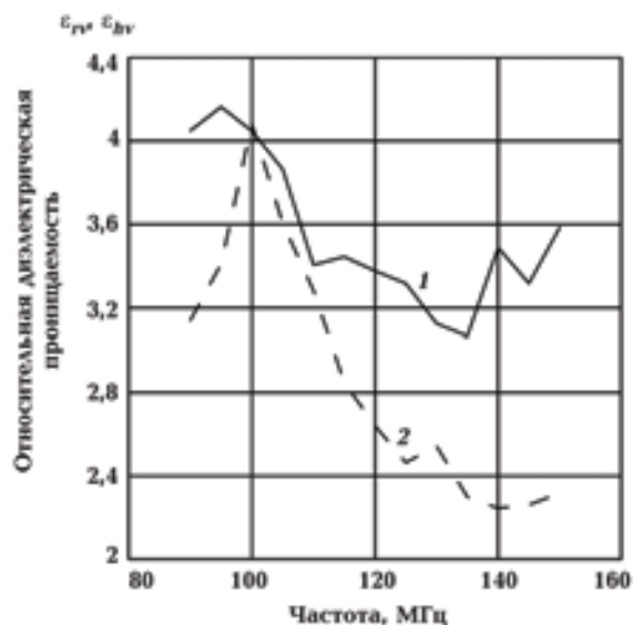
Рис. 5. Диэлектрическая проницаемость образца влажного песка под давлением: 1 — вертикальный датчик, 2 — горизонтальный датчик.
