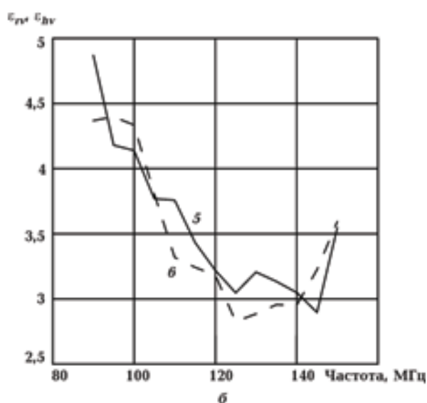
Рис. 9. Диэлектрическая проницаемость влажного песка без давления (кривые 1, 2) и после приложения давления (кривые 3, 4) (а), а также после снятия давления (кривые 5 и 6) (б).
