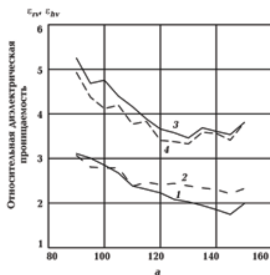
Рис. 9. Диэлектрическая проницаемость влажного песка без давления (кривые 1, 2) и после приложения давления (кривые 3, 4) (а), а также после снятия давления (кривые 5 и 6) (б).
