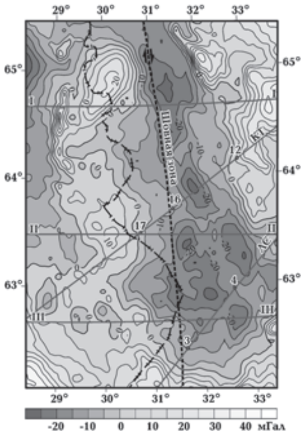
Рис. 2. Гравитационное поле (аномалии Буге) центральной части Карельского крагона и положение профилей ГСЗ (КТ — Кемь—Тулос, АС — Лахденпохья—Сегозеро) с пунктами взрыва и интерпретационных профилей I—I, II—II, III—III. Условные обозначения см. на рис. 1.
