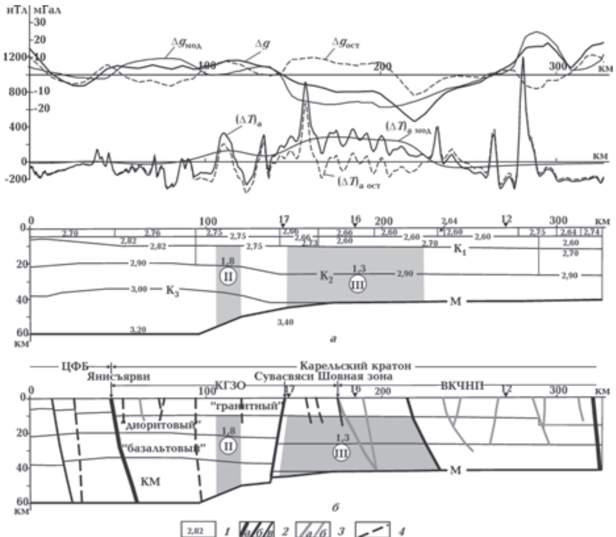
Рис. 12. Плотностная и магнитная модели (а) и их структурная интерпретация (б) по профилю ГСЗ Кемь—Тулос: 1 — значения плотности, \text{г/см}^3 , 2 — система разломов (а—I, б—II, в—III рангов северо-западного простирания), 3 — система разломов меридионального шва (а—II, б—III рангов), 4 — разломы других направлений, в том числе дугообразные. КГЗО — Карельская гранит-зеленокаменная область, ВКЧНП — Восточно-Карельский чешуйчато-надвиговый пояс, KM — коромангийная смесь, M — граница раздела Мохоровичича. Положение профиля и другие условные обозначения см. на рис. 3, 4.
