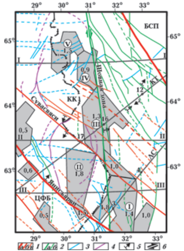
Рис. 21. Трехмерная магнитная модель средней и нижней коры центральной части Карельского кратона: 1 — система разломов северо-западного простирания ( a — I, b — II, v — III рангов); 2 — система разломов меридионального шва ( a — II, b — III рангов); 3 — разломы других направлений; 4 — дугообразные разломы; 5 — направления падения разломов; 6 — направления горизонтальных перемещений. БСП — Беломорский складчатый пояс. Разрывные нарушения (сплошные линии — разломы, выделенные по геологическим данным, пунктирные — по магнитному и гравитационному полям). Другие условные обозначения см. на рис. 2, 3.
