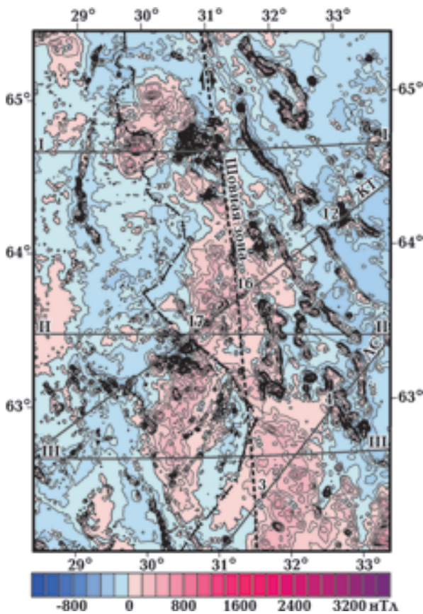
Рис. 18. Аномальное магнитное поле ( \Delta T_a ) центральной части Карельского кратона (изолинии в нТл). Другие условные обозначения см. на рис. 2.
