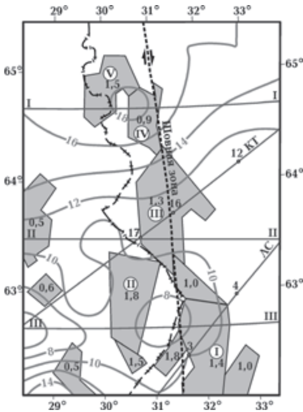
Рис. 4. Схема глубины залегания границы K_1 (км) и положение верхних кромок источников региональных магнитных аномалий (РМА). Другие условные обозначения см. на рис. 2, 3.
