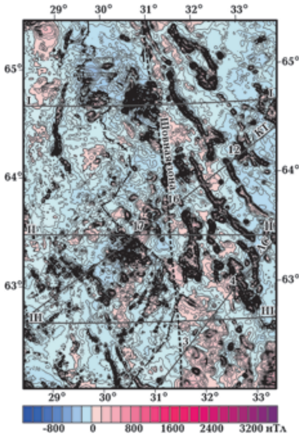
Рис. 20. Разностное поле ( \Delta T_a ), нТл. Другие условные обозначения см. на рис. 2.
