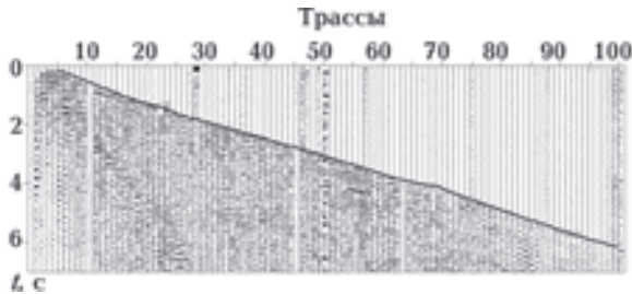
Рис. 9. Корреляция годографа по волновому полю для SP01.
