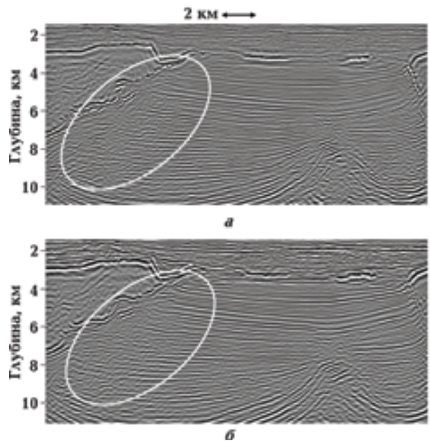
Рис. 10. Сейсмические изображения, полученные в Мексиканском заливе после применения миграции в обратном времени с VTI (а) и ТТИ (б) моделью скоростной анизотропии.
