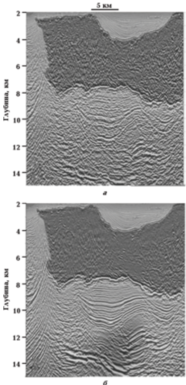
Рис. 1. Сейсмические изображения, полученные в Мексиканском заливе после применения миграции одностороннего волнового уравнения до (а) и после (б) уточнения скорости под солью с помощью лучевой томографии.
