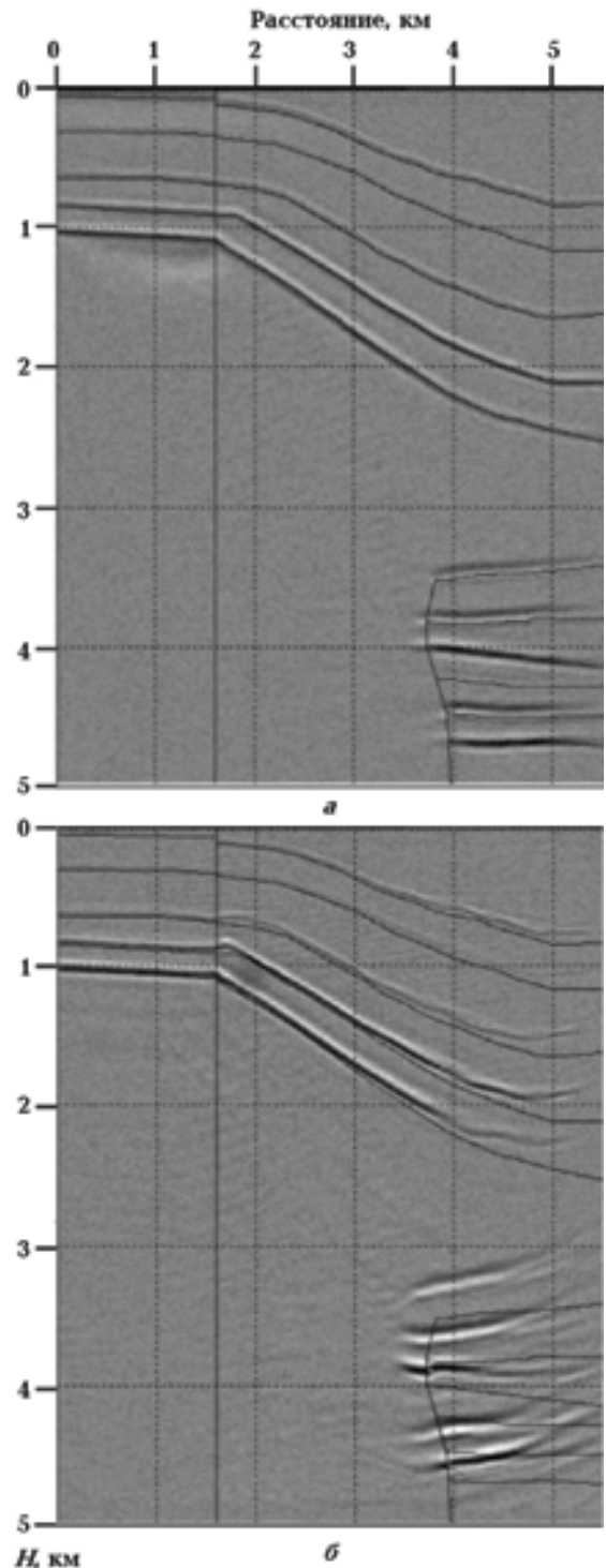
Рис. 8. Сейсмические изображения, полученные с учетом (а) и без учета (б) анизотропии скоростей по синтетическим данным, соответствующим модели, изображенной на рис. 7.
