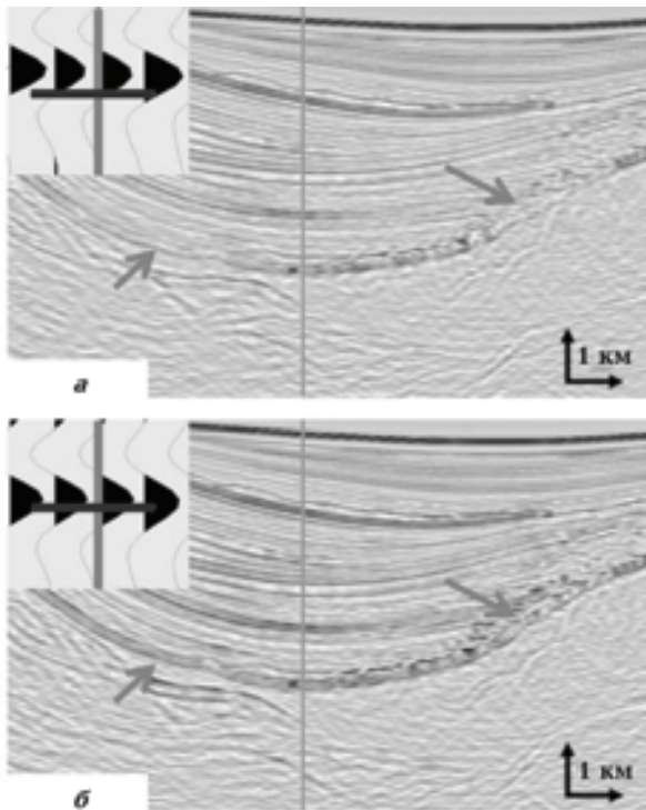
Рис. 13. Сейсмические изображения, полученные со скоростными моделями ТТИ (а) и T-ORT (б) в Мексиканском заливе. Траектория скважины обозначена вертикальной линией. Отклонения обоих изображений от маркера кровли соли в скважине (горизонтальная линия) показаны в увеличенном масштабе. Они равны 20 и 8 м после миграций с моделями ТТИ и T-ORT соответственно.
