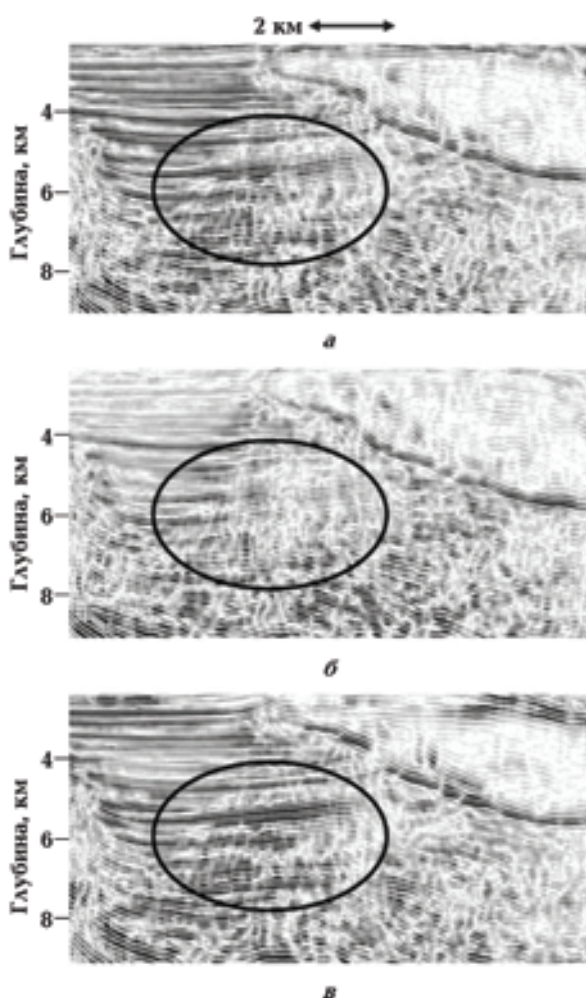
Рис. 2. Результаты миграции в обратном времени в Мексиканском заливе при различных временных задержках изображения: 0 мс (а), 100 мс (б) и – 100 мс (в).
