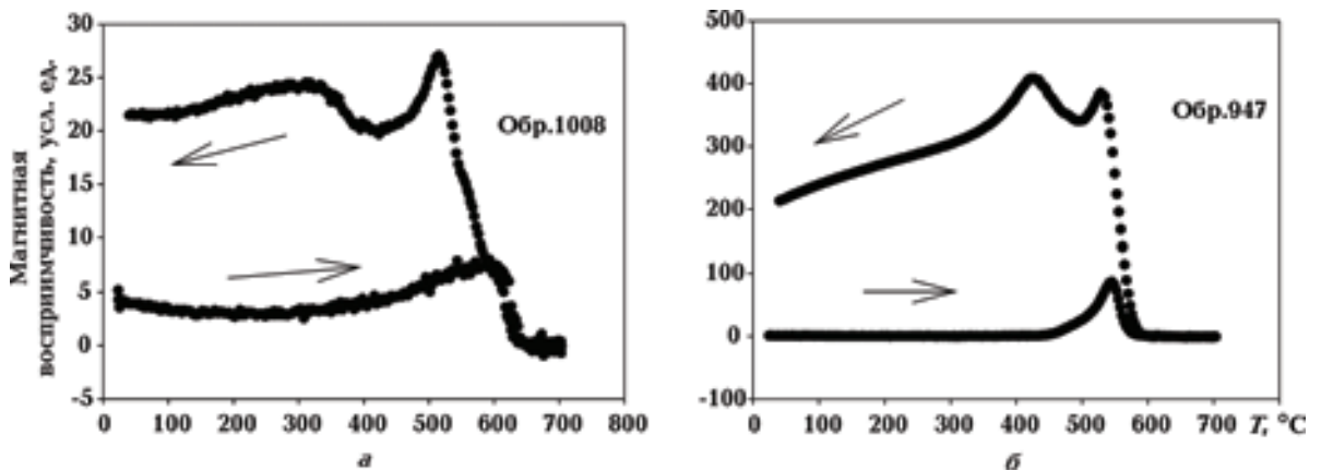
Рис. 7. Изменение магнитной восприимчивости образцов красцветов в процессе непрерывного нагрева и охлаждения.
