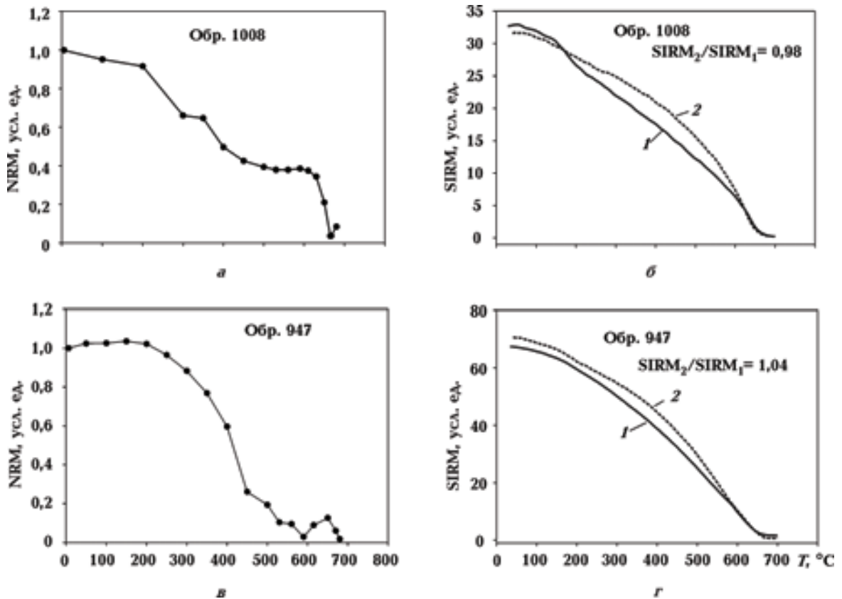
Рис. 6. Примеры температурного размагничивания образцов красцветов: нормированной NRM в процессе ступенчатого размагничивания (а, в); остаточной намагниченности насыщения (SIRM) в процессе непрерывного нагрева (1 — первый нагрев, 2 — второй нагрев) (б, г).
