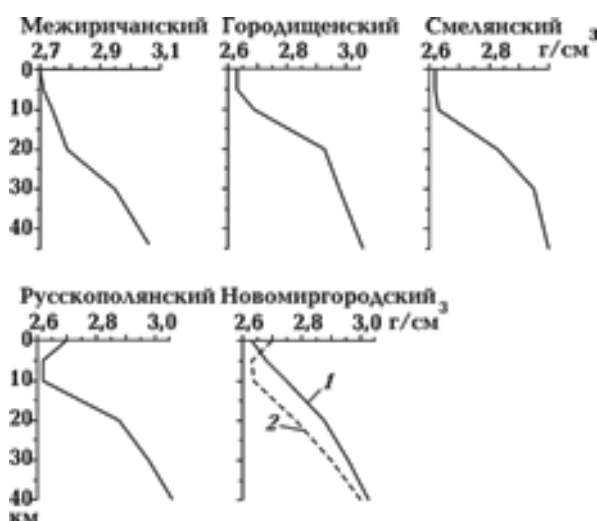
Рис. 10. Изменение плотности с глубиной в массивах габбро-анортозитов. Расположение точек см. на рис. 1.
