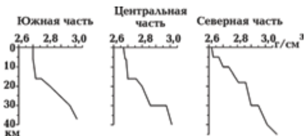
Рис. 12. Изменение плотности с глубиной на площади развития биотитовых гнейсов. Расположение точек см. на рис. 1.
