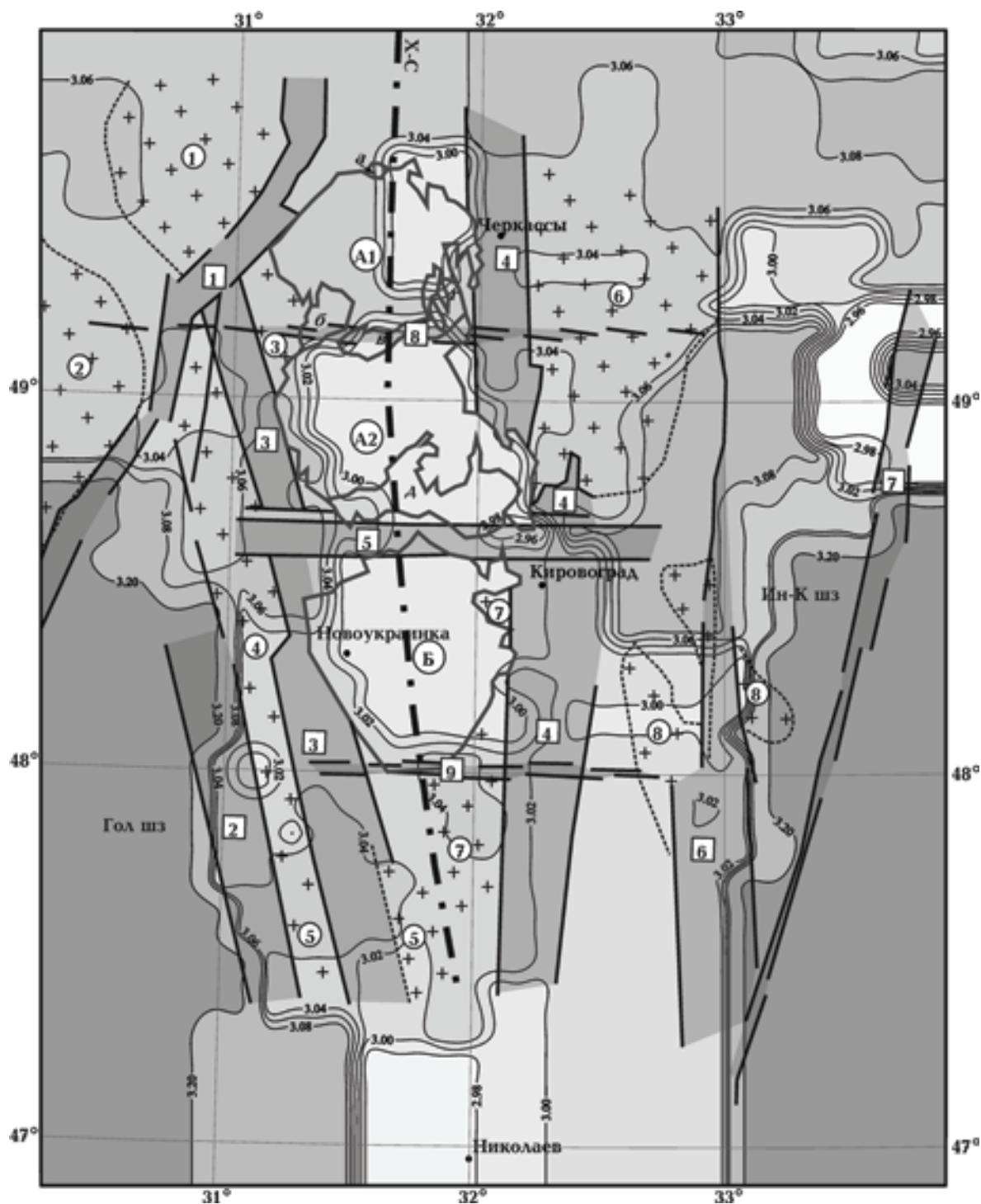
Рис. 8. Схема распределения плотности ( \text{г/см}^3 ) на поверхности Мохо. Условные обозначения см. на рис. 1.
