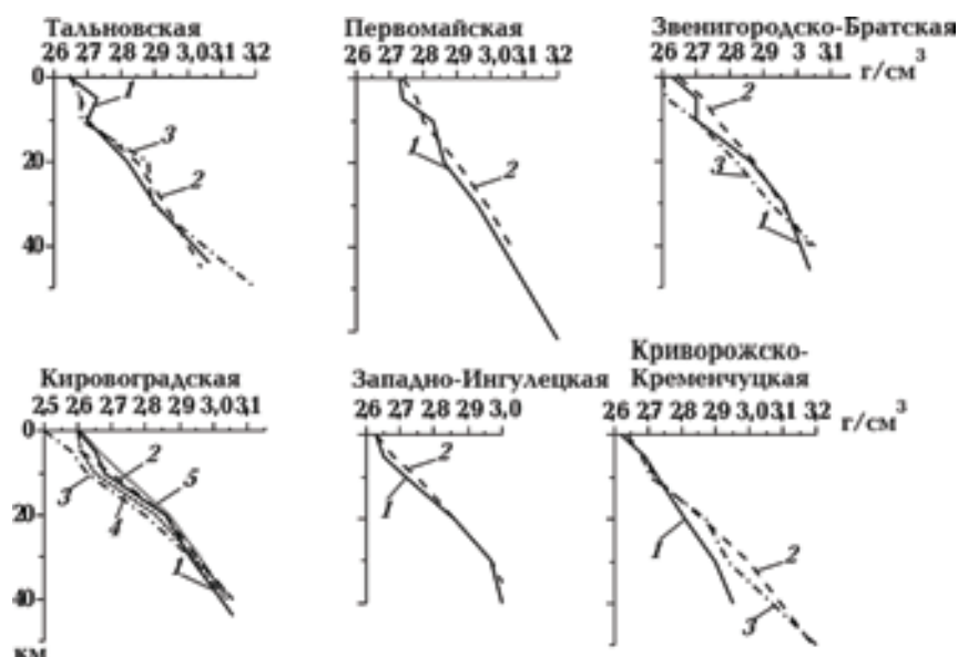
Рис. 14. Изменение плотности с глубиной в зонах разломов. Расположение точек см. на рис. 1.
