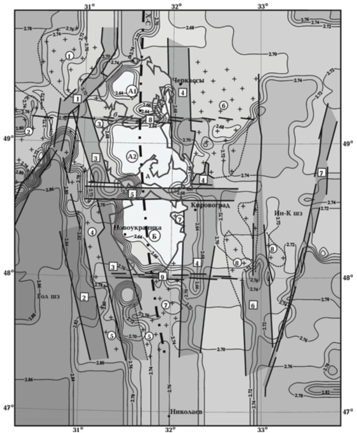
Рис. 5. Схема распределения плотности ( \text{г/см}^3 ) на глубине 10 км. Условные обозначения см. на рис. 1.
