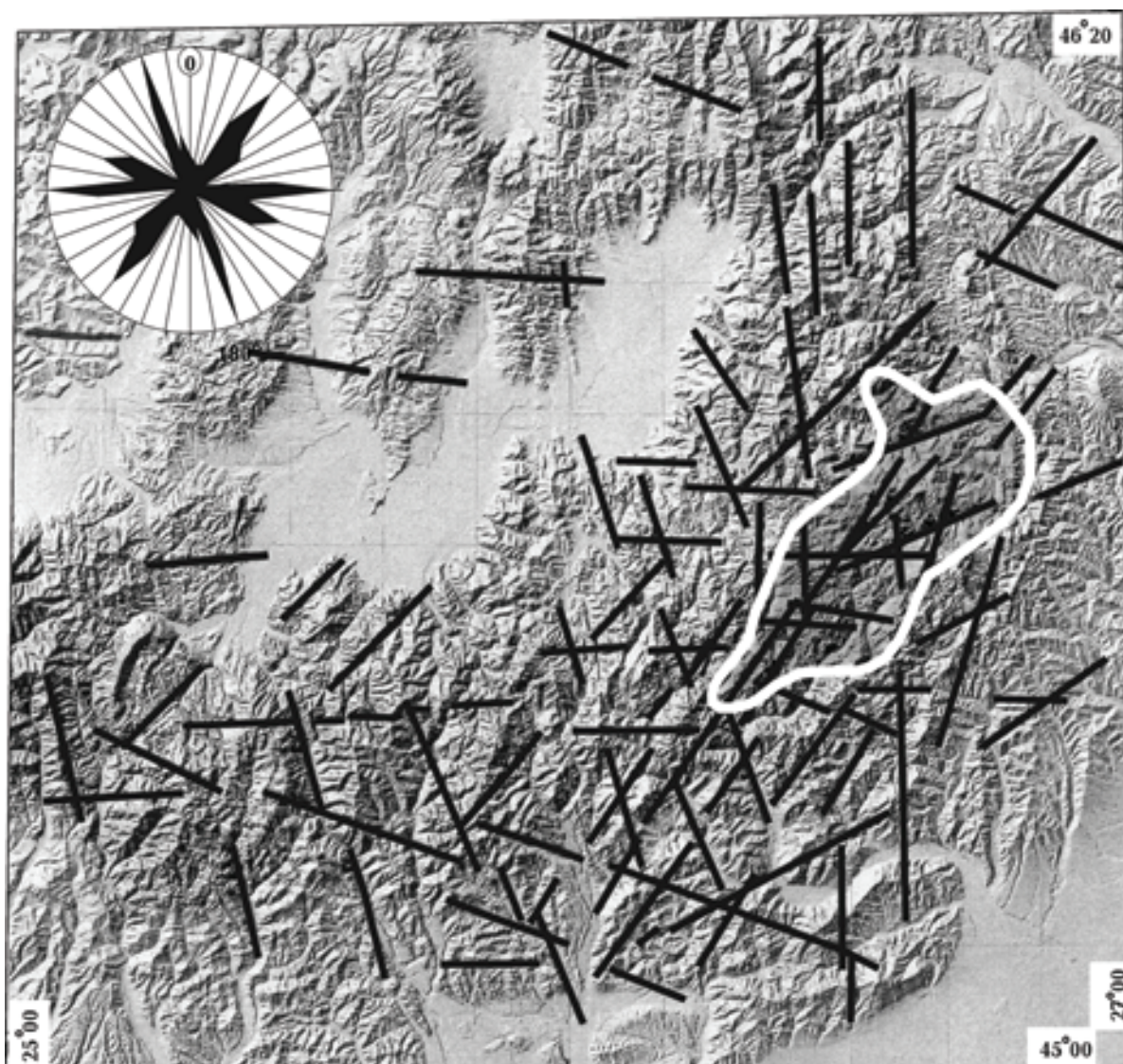
Рис. 6. Карта 3D рельефа района исследований. Белым контуром обозначена среднеглубинная сейсмогенная ЗВ; прямолинейные отрезки соответствуют тополинаментам, азимуты простирания которых обобщены на розе-диаграмме (врезка).
