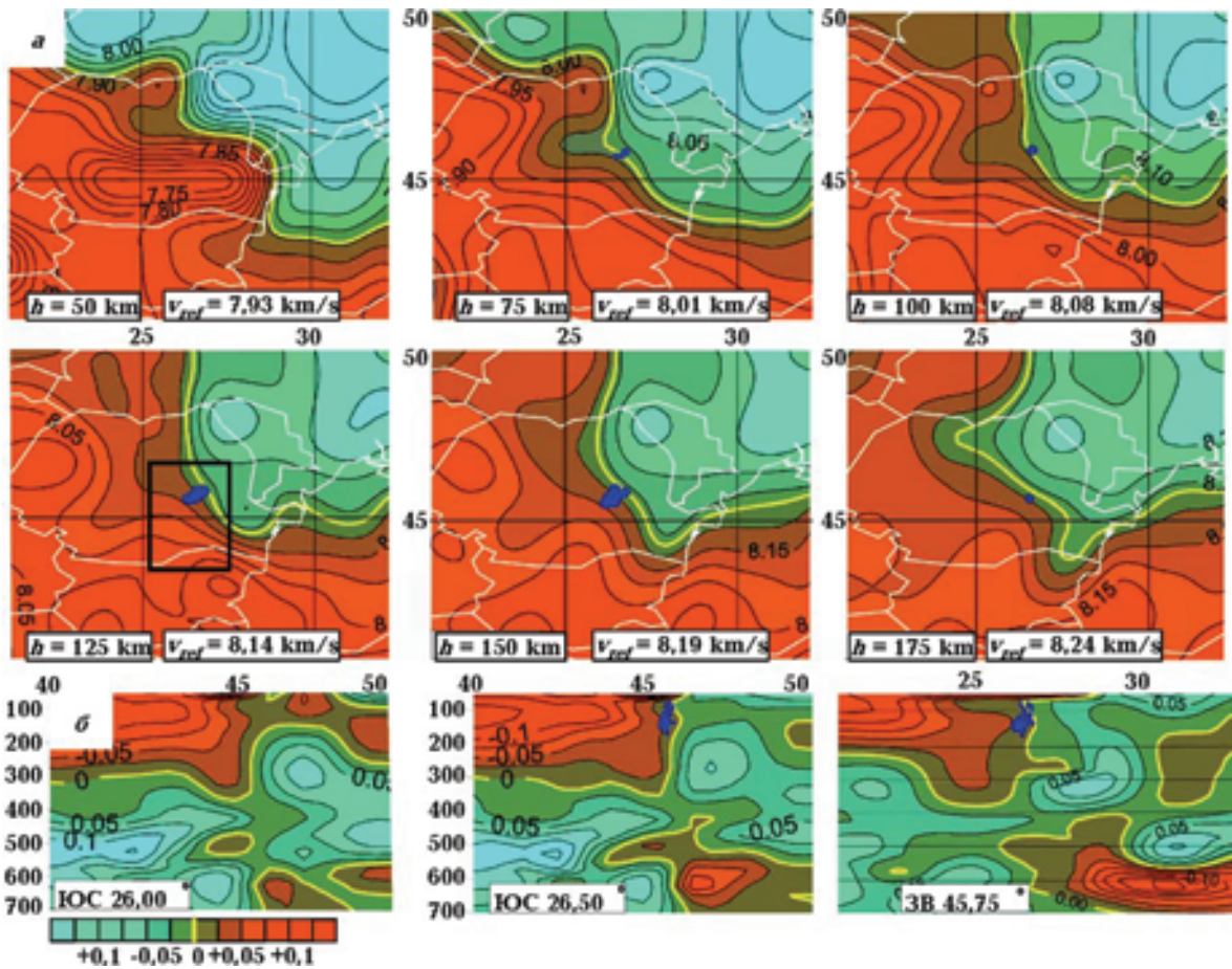
Рис. 8. Региональные сейсмотомографические сечения района исследования, по [Старостенко и др., 2013]: а — горизонтальные ( V_p , км/с), б — вертикальные ( \Delta V_p , км/с). Прямоугольником отмечена площадь детальных сейсмотомографических исследований, по [Koulakov et al., 2010].
