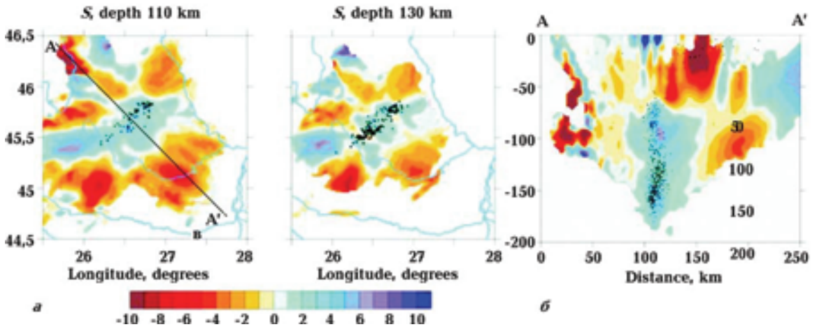
Рис. 9. Локальные сейсмотомографические сечения зоны Вранча, по [Koulakov et al., 2010]: а — горизонтальные, б — вертикальное.
