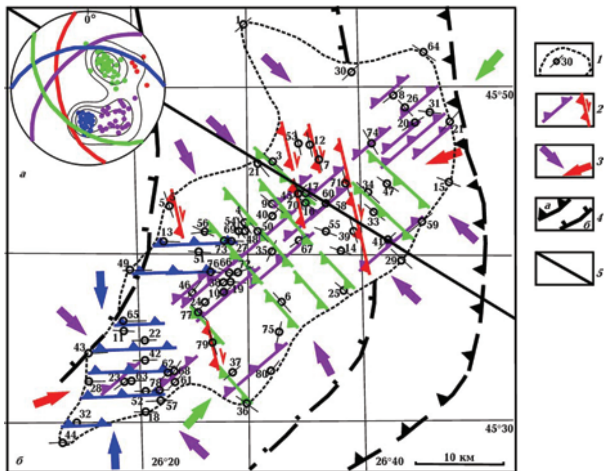
Рис. 3. Результаты тектонофизической интерпретации механизмов очагов землетрясений ЗВ: а — стереограмма полюсов нодальных площадок и обобщенных плоскостей, соответствующих (по цвету) максимумам концентрации полюсов (нижняя полусфера); б — обобщенный структурный план ЗВ для глубины 80—170 км: 1 — граница зоны, эпицентры землетрясений с номерами и простирание действующих нодальных площадок, 2 — зоны концентрации нодальных площадок соответствующих направлений с указанием направлений падения и сдвигового перемещения, 3 — направления субгоризонтального сжатия для соответствующих (по цвету) зон концентрации нодальных площадок, 4 — границы ( а — Флишевых Карпат, б — отдельных покровов), 5 — линия сейсмического профиля Вранча-2001.
