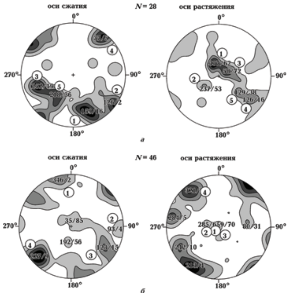
Рис. 5. Стереогаммы (нижняя полусфера) осей максимального и минимального сжатия для: а — Восточных (район Команешти—Онешти), б — Южных (район Калиманешти—Титешти) Карпат, по [Manenco et al., 1997 a, b]. Цифры в кружках — номера максимумов концентрации осей. Белые дроби — обобщенные азимут/угол наклона осей.
