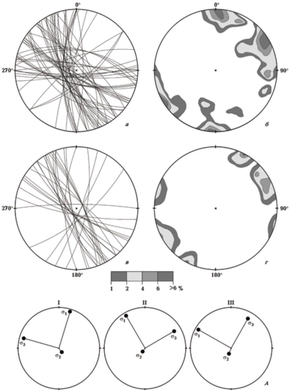
Рис. 3. Структурные S - и \pi S -диаграммы для трещин скалывания (а, б) и отрыва (в, г), а также поля напряжений поздних стадий развития зоны ЗГР (д); \sigma_1 — ось максимального сжатия; \sigma_2 — ось промежуточных напряжений; \sigma_3 — ось максимального растяжения.
