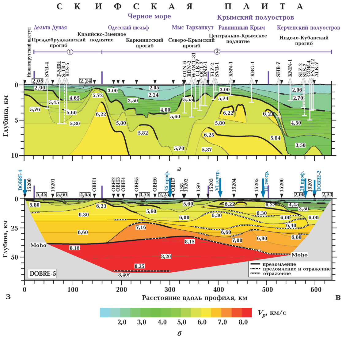
Рис. 3. Двумерная сейсмическая модель: а — по скоростям распространения продольных волн вдоль профиля DOBRE-5 в осадочном чехле: цифры в кружках : 1 — Предбурджанский сегмент; 2 — Крымско-Азовский сегмент Скифской плиты); полученная по методу лучевого (ray-tracing) моделирования коры и верхней мантии с использованием программного пакета SEIS83 [Starostenko et al., 2015]. Черными линиями обозначены скоростные границы, толстыми черными линиями — преломленные или/и отраженные границы. Тонкими линиями показаны изолинии скоростей и их значения (в км/с) в белых прямоугольниках, черными стрелками — положение пунктов взрывов; голубыми стрелками — пересечения с другими профилями. Вертикальный масштаб: ~14,5:1 — для осадочного чехла модели; ~2,4:1 — для полной модели. Скважины (данные производственных организаций): SVR-4 — Суворовская (13,2 км на север от профиля); FMR1 — Фурмановская (5,7 км на север); S-TR-1 — Старотрояновская (28,5 км на север); KLS-5 — Килийская (16,0 км на север); OLN-6 — Оленевская (2,8 км на юг); RDN-2 Родниковская (0,8 км на юг); W-ОСТ-31 — Западно-Октябрьская (1,6 км на юг); GLB-27 — Глебовская (9,6 км на север); ОСТ-2 — Октябрьская (2,8 км на юг); DNZ-1 — Донузлавская (5,0 км на север); ELZ-2 — Елизаветинская (0,6 км на юг); SVR-1 — Северская (7,2 км на север); KSN-3 — Донусовская (5,8 км на север); KRG-1 — Красногвардейская (12,6 км на север); SHB-7 — Шубинская (1,6 км на север); KMN-1 — Каменская (1,4 км на север); SLZ-2 — Селезневская (2,0 км на север); SLS-2 — Слюсаревская (1,6 км на юг); GOR-4 — Горностаевская (3,1 км на север); FNT-12 — Фонтановская (0,4 км на север); ALK-7 — Алексеевская (0,4 км на север).
