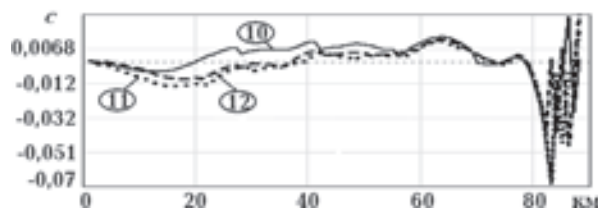
Рис. 9. Невязка между референц-географом и моделируемым после 10, 11 и 12 тысяч итераций.
