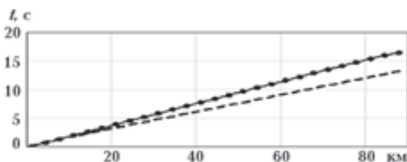
Рис. 3. Годографы на трассе в 88 км: пунктиром показан годограф, генерируемый первичной скоростной функцией рис. 2, сплошной линией — наблюдаемый референц-годограф, точками — «отожженный» годограф после 10 тысяч итераций.
