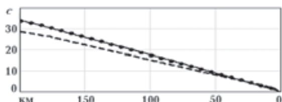
Рис. 13. Сборка годографов профиля длиной 187 км: пунктир — годограф стартовой скоростной функции, сплошная — референц-годограф, точки — годограф после 10 тысяч итераций.
