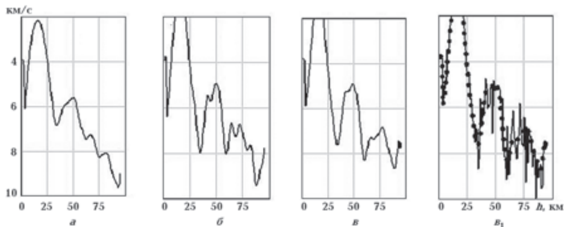
Рис. 17. «Отожженная» скоростная функция после 8 (а), 9 (б) и 10 тысяч итераций (в); сплошной линией ( v_1 ) показан выход скоростной функции рисунка в (точка — кривая).
