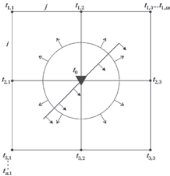
Рис. 1. Схема участка сеточной области, содержащего источник колебаний, фронты локальной плоской и сферической волн.
