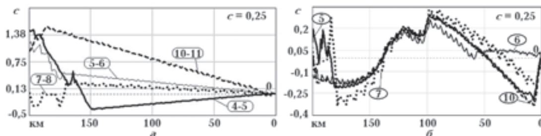
Рис. 15. Векторы невязок годографов: а — невязки, вызванные фильтрацией функции скорости для тысяч итераций, показанных в овалах; б — невязки референц-годографа с таковым, полученным в результате отжига для количества итераций, приведенных в овале.
